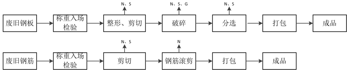
图 5-1 工艺流程图
